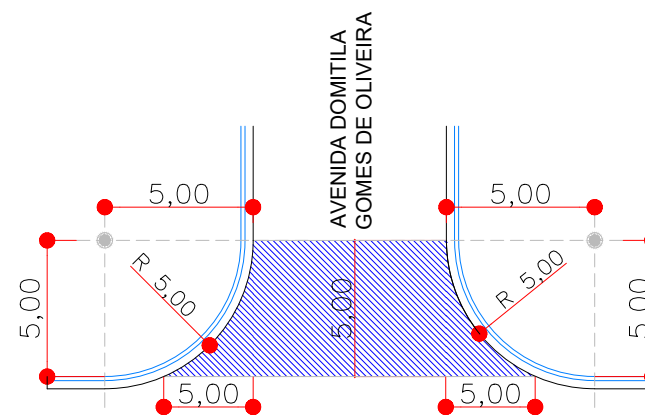
ÁREA DE UM LIMPA-RODAS A=66,9801 m 2 de uma limpa-rodas RUA CICERO SAMPAIO DE MENESES
