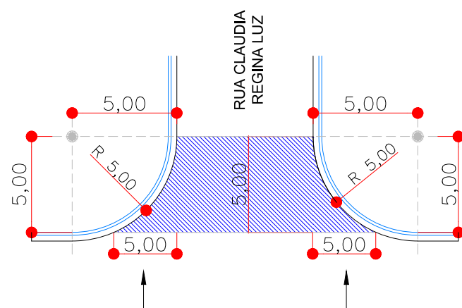
ÁREA DE UM LIMPA-RODAS A=50,7301 m 2 de uma limpa-rodas A=50,7301 m 2 de uma limpa-rodas AVENIDA ROBENS R. ARAUJO FILHO
