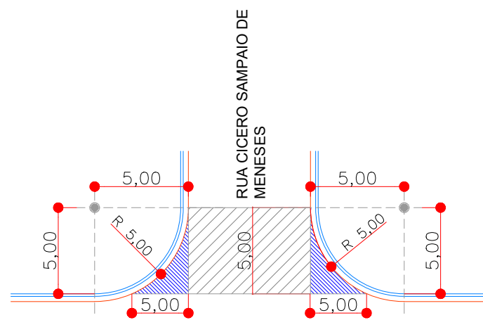
ÁREA DE EMBOCADURA A=11,4867m 2 de uma Embocadura AVENIDA DOMITILA GOMES DE OLIVEIRA
