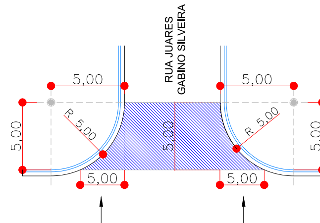
ÁREA DE UM LIMPA-RODAS A=50,7301 m 2 de uma limpa-rodas A=50,7301 m 2 de uma limpa-rodas AVENIDA ROBENS R. ARAUJO FILHO
