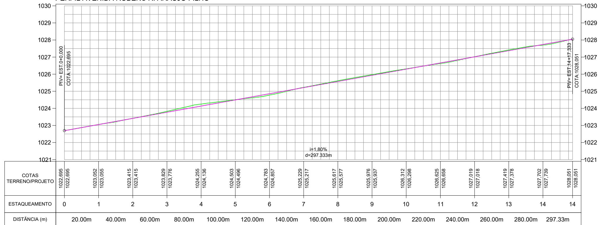
PERFIL AVENIDA ROBENS R. ARAUJO FILHO
