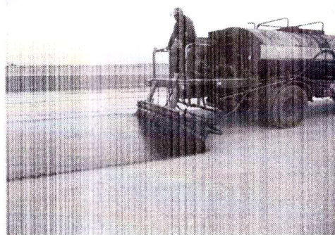
Execução de imprimação
