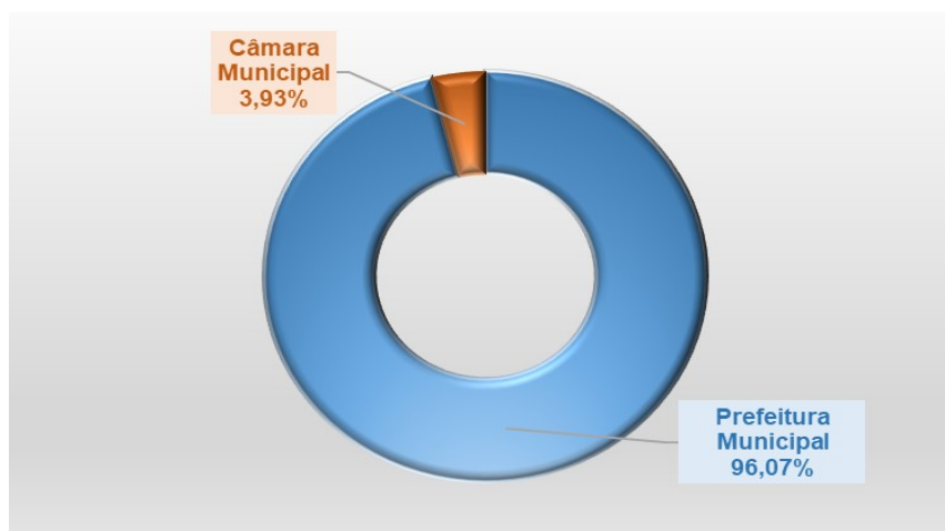
Gráfico 1 – Distribuição Orçamentária
