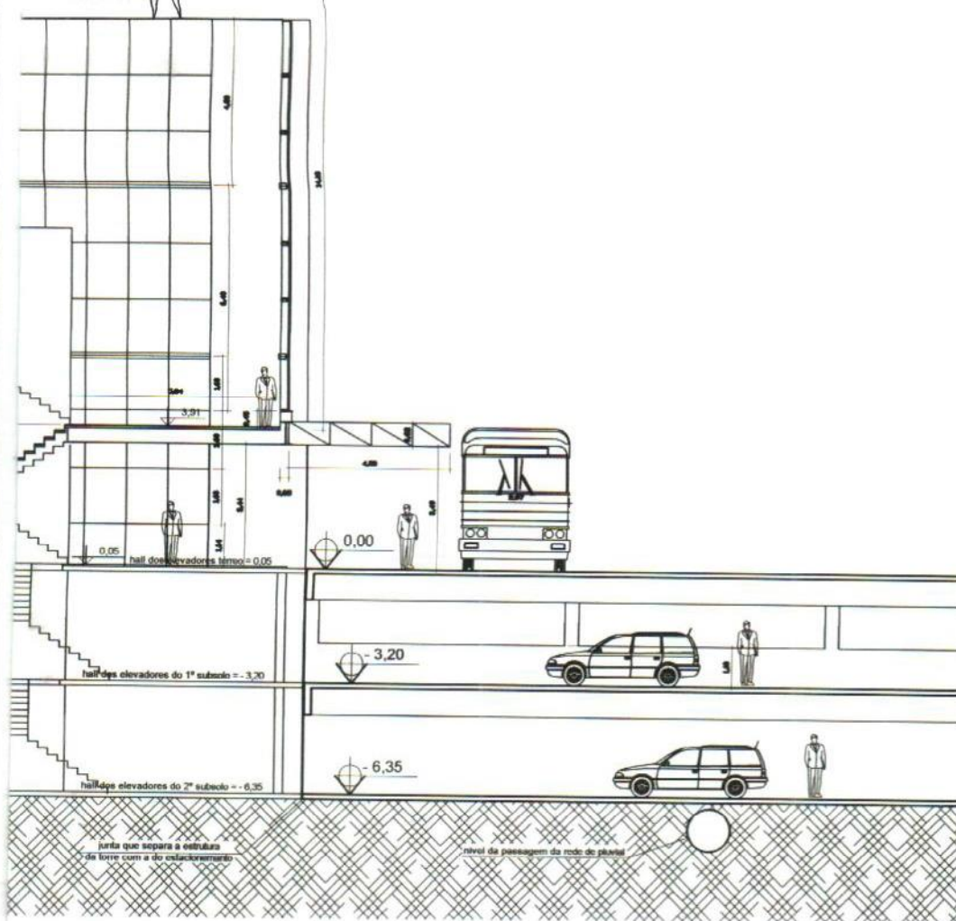
CORTE AA
