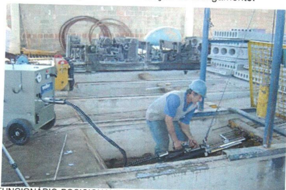
FIGURA 7 – FUNCIONÁRIO POSICIONANDO O MACACO QUE PROTENDE CADA CORDOALHA ISOLADAMENTE. FONTE: PETRUCELLI (2009).
